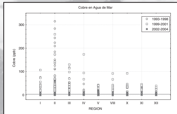
Figura 6.18: Cobre en Agua
